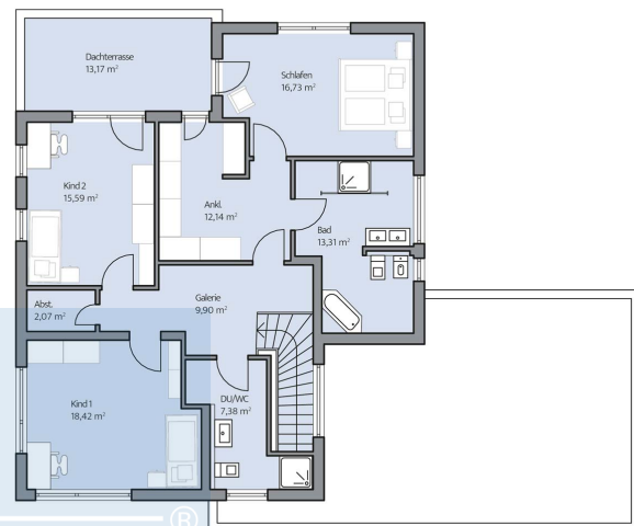
Haus Schoenborn Grundriss
