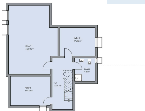
Haus Schoenborn Grundriss
